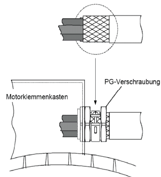
EMV-gerechter Motoranschluss
