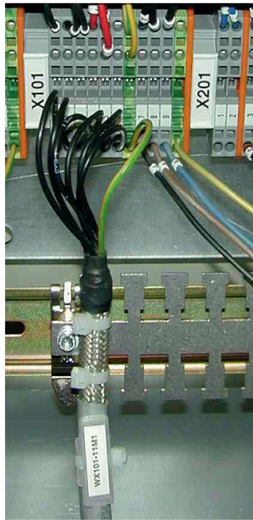
Kabelschirmung_Foto mit Kabelbindern
