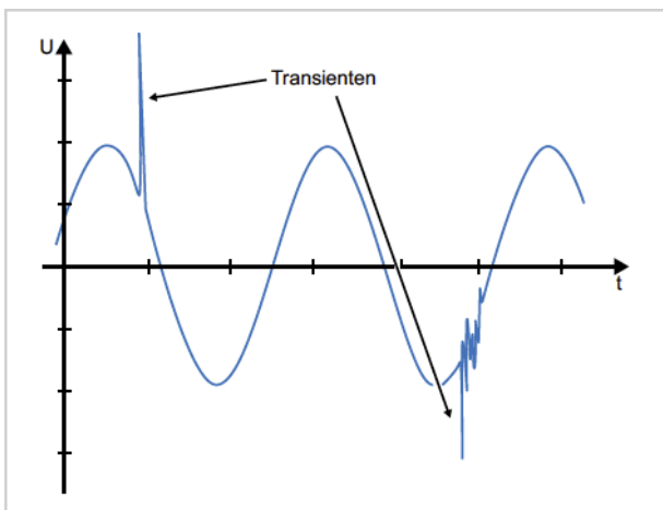
Transienten (Spannungsspitzen)
